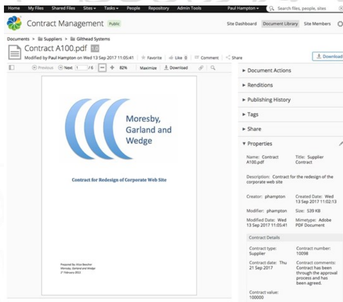
Figura 7: Ejemplo de un documento disponible en un repositorio Alfresco. Puede verse el documento, junto con sus metadatos. Imagen obtenida de: https://en.wikipedia.org/wiki/Alfresco_Software .
